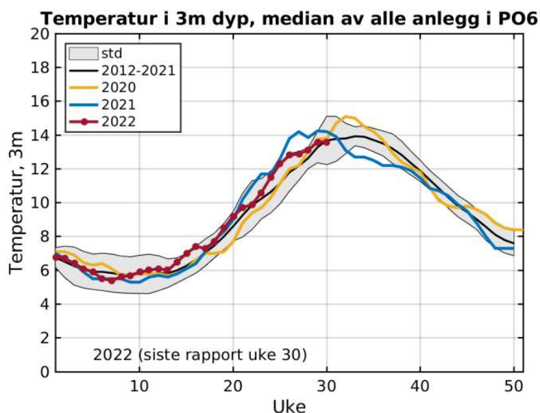
Figur 1: Observert temperatur i 3m dyp. Sort linje viser middelveiden (2012-2021) og skravert felt viser pluss/minus et standardavvik.
